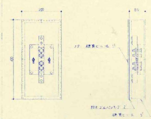
接地鋼板 (無錫ロ付)
