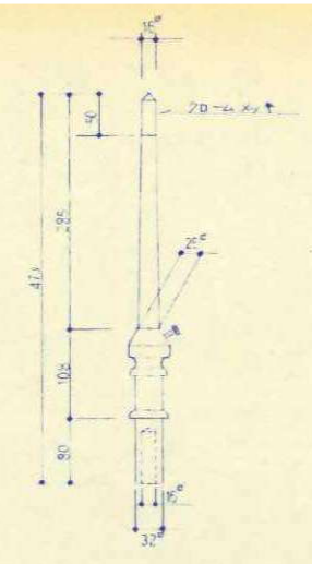
試験用端子並:建設者TB-CSIA 硬樹脂 (露出型)
