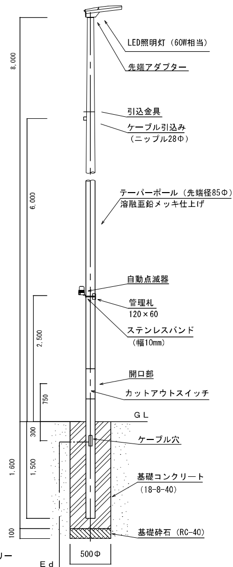
独立柱共架図
