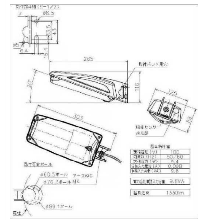
寸法図
