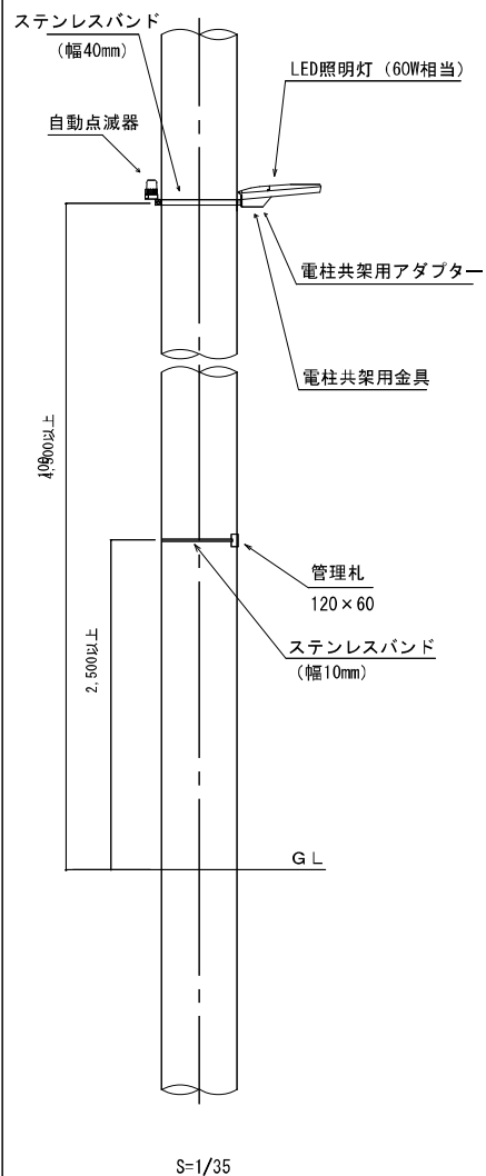
電柱共架図
