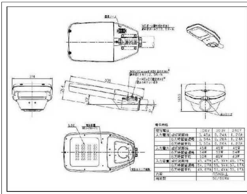
寸法図 (参考)
