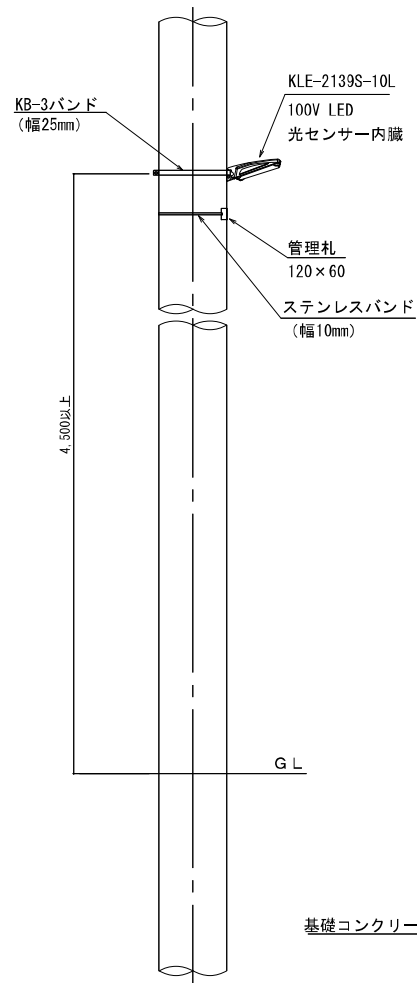
電柱共架図
