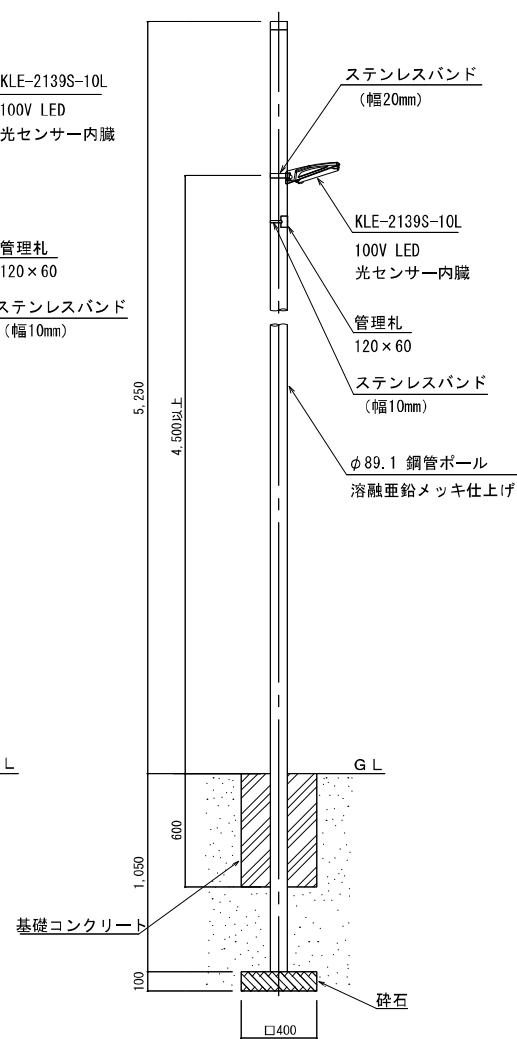
ポール共架図
