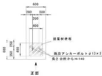
アンカー位置図
