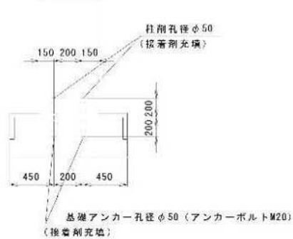
アンカー位置図
