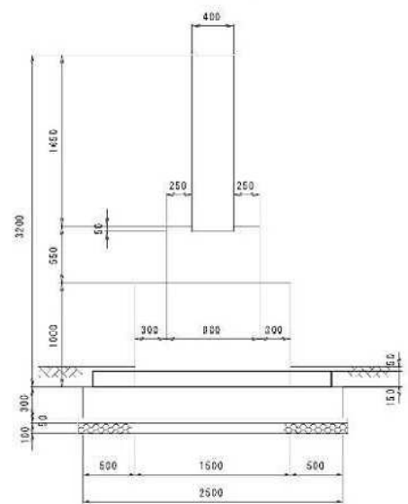
アンカー位置図
