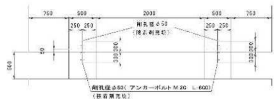
アンカー位置図
