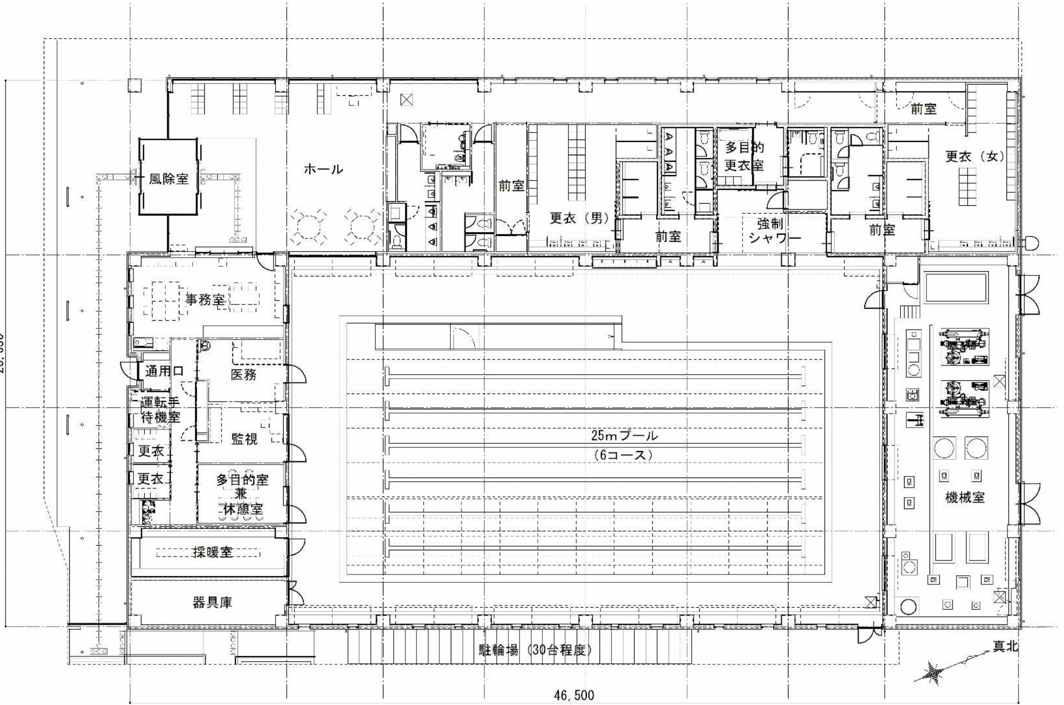
平面図
